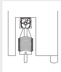
Monté dans le linteau
